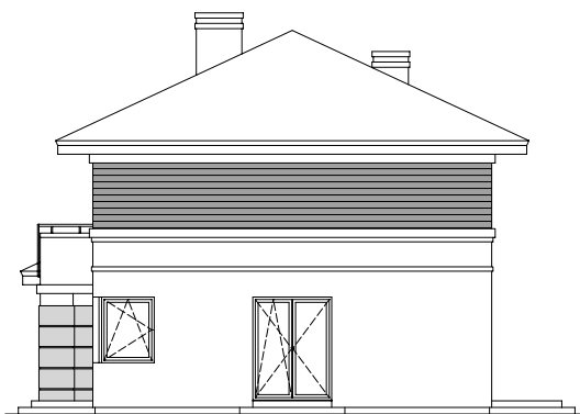
ELEWACJA PRAWA
