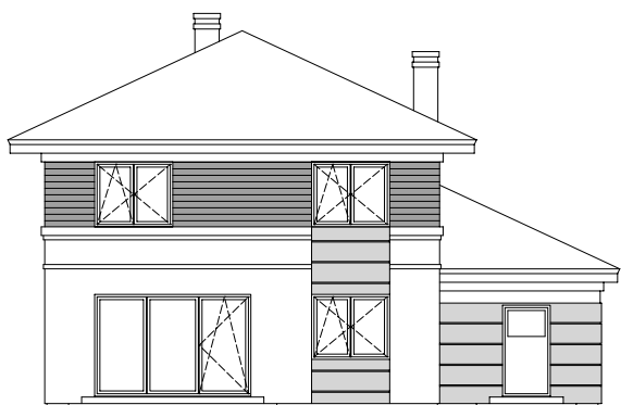
ELEWACJA OGRODOWA
